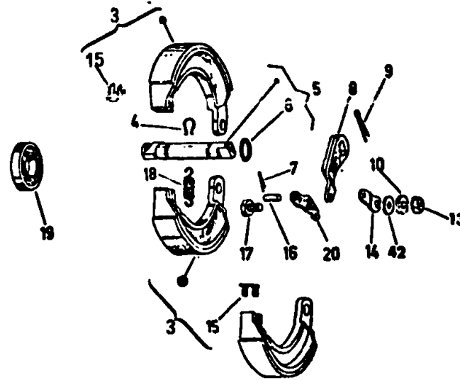
Hinterradnabe - Schaltgetriebe
